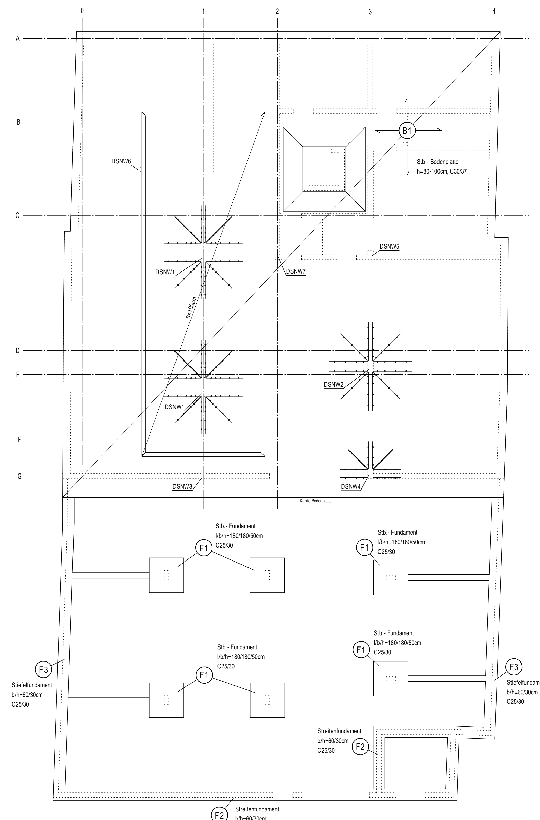
Gründung
