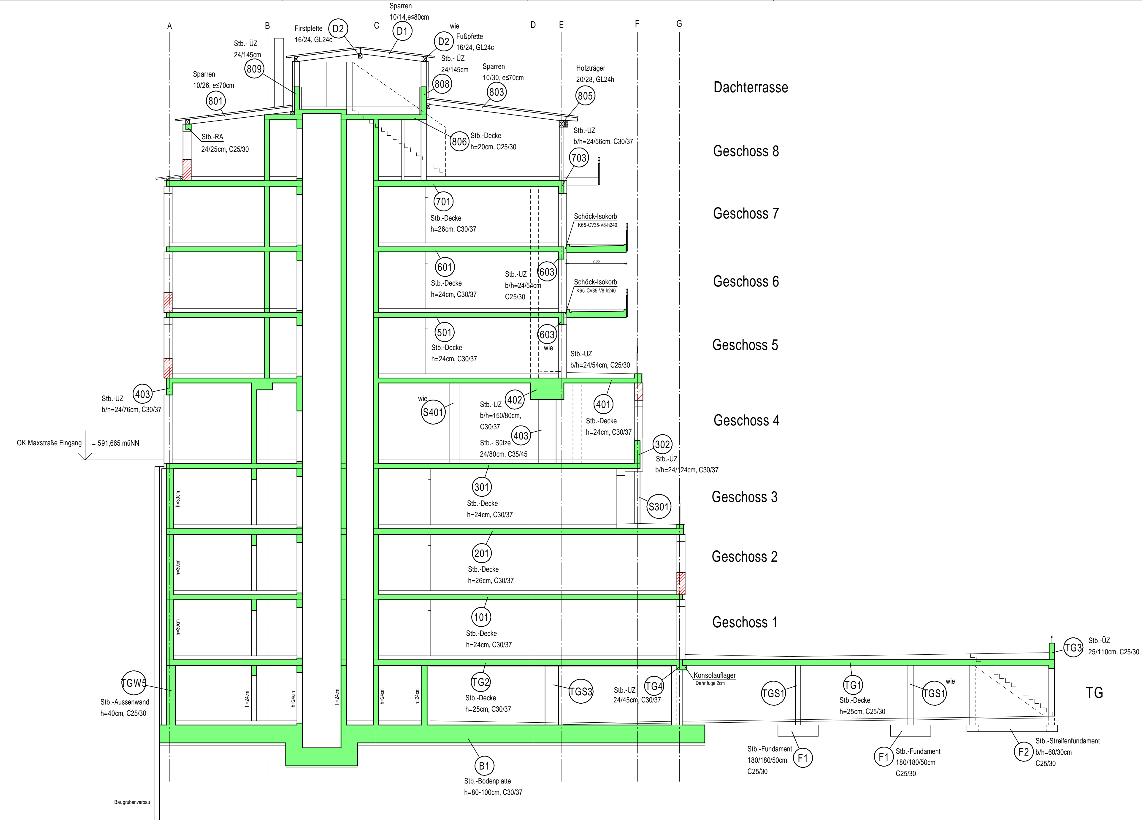
Gründung
