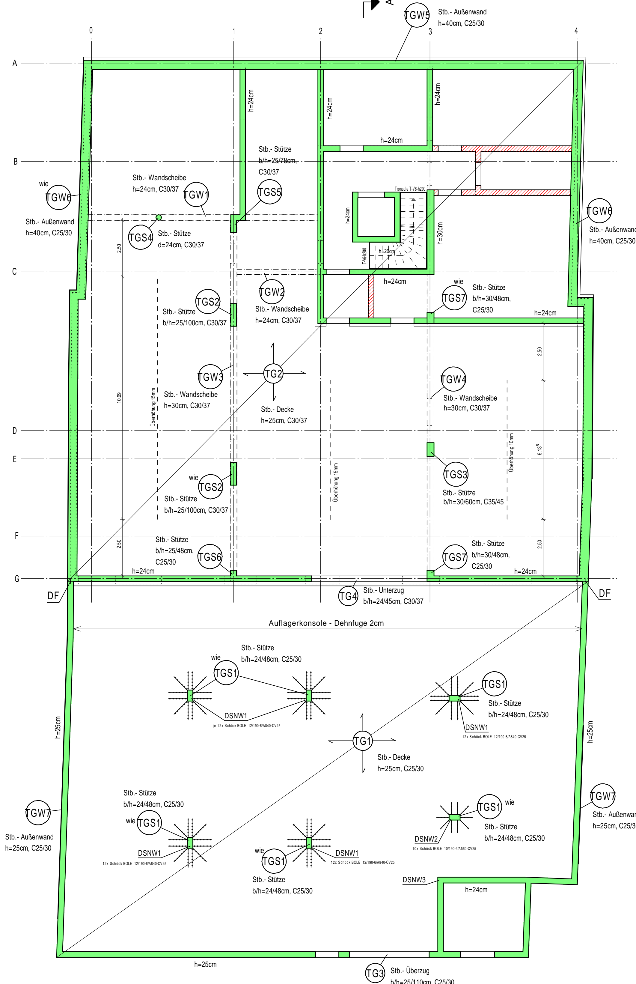
Tiefgarage
